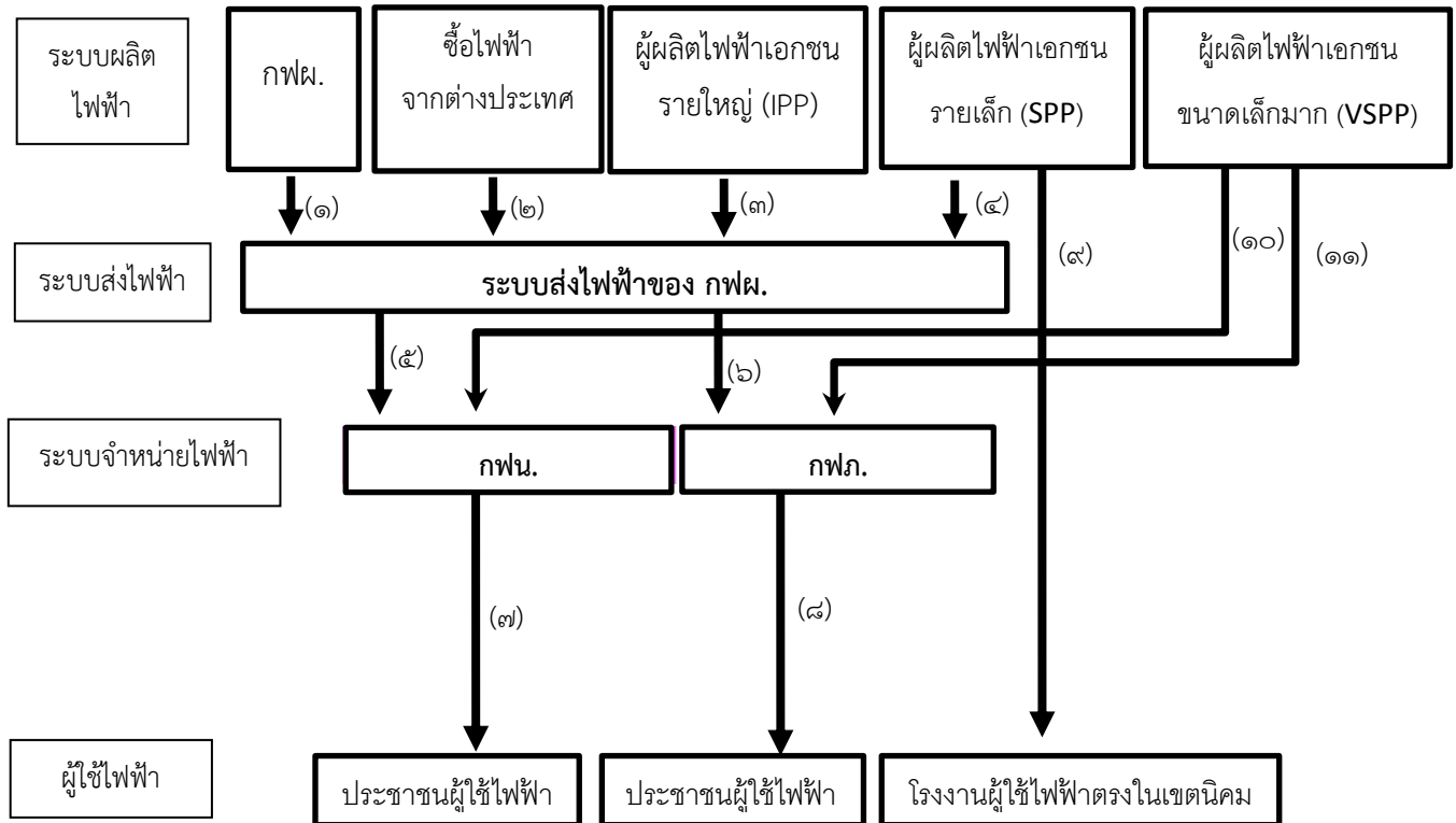
รูปภาพที่ ๑ ลักษณะของกิจการไฟฟ้าของประเทศไทยในปัจจุบันซึ่งเป็นระบบผู้ซื้อไฟฟ้ารายเดียว (Enhanced Single Buyer) ในรูปแสดงการขายพลังงานไฟฟ้าจากผู้ผลิตไปสู่ผู้ซื้อไฟฟ้า
